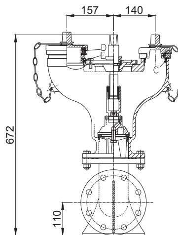
地下消火栓 SA100/65-1.6
