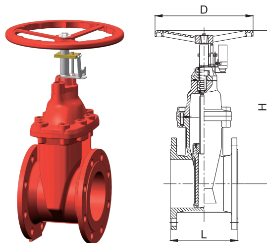
FIG. F0255, 法兰X法兰
